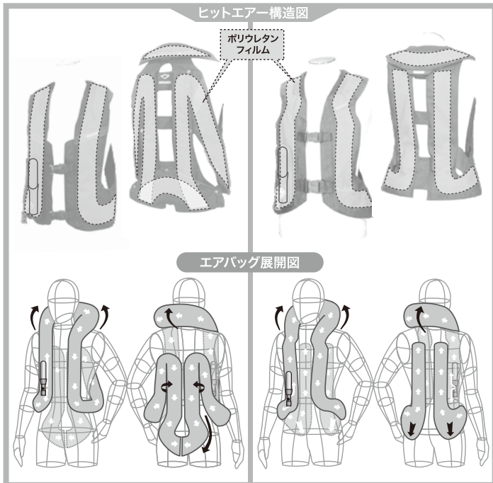
ヒットエア―ー構造図
